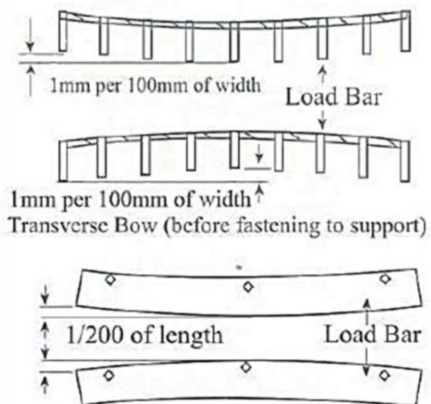
Longitudinal Bow
